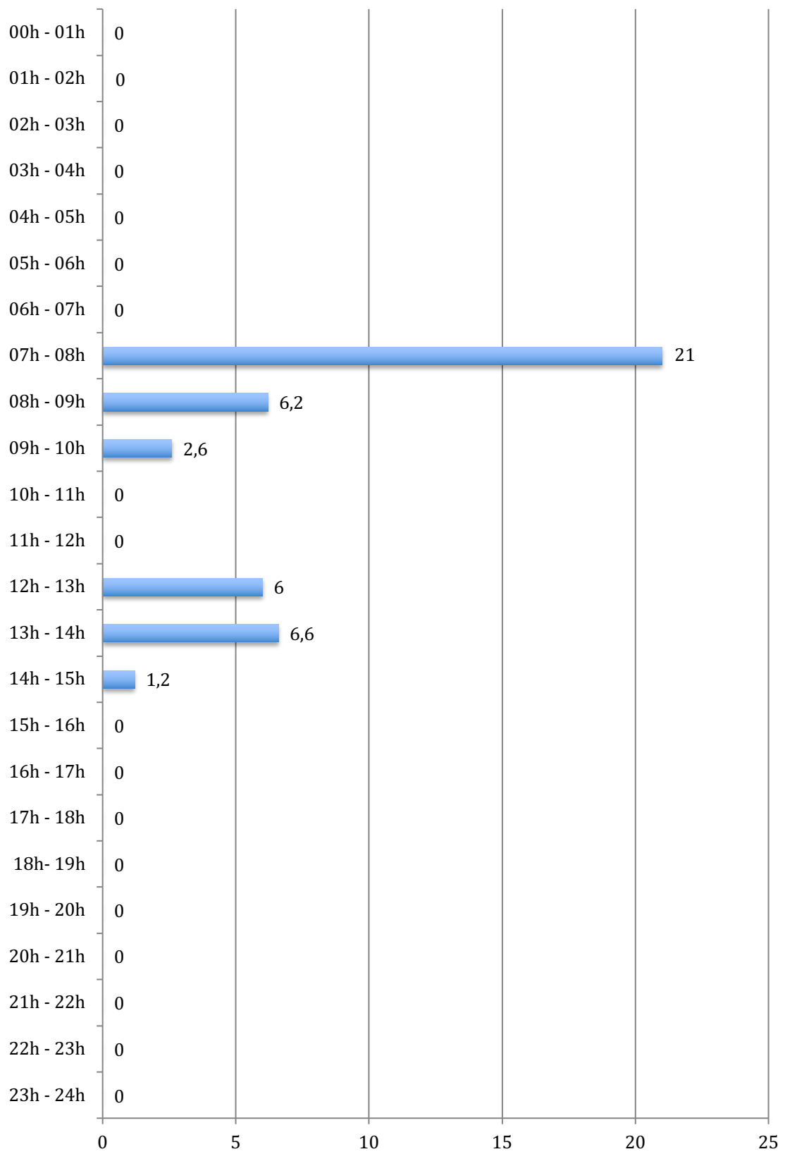
Cantidades de lluvia registradas por horas en EL REAL DE GANDÍA el día 16/05/20 (en l/m²)
