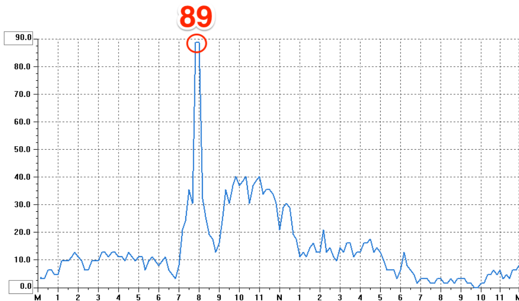
Ráfagas de viento registradas en EL REAL DE GANDÍA el sábado 16/05/20 (en km/h)
